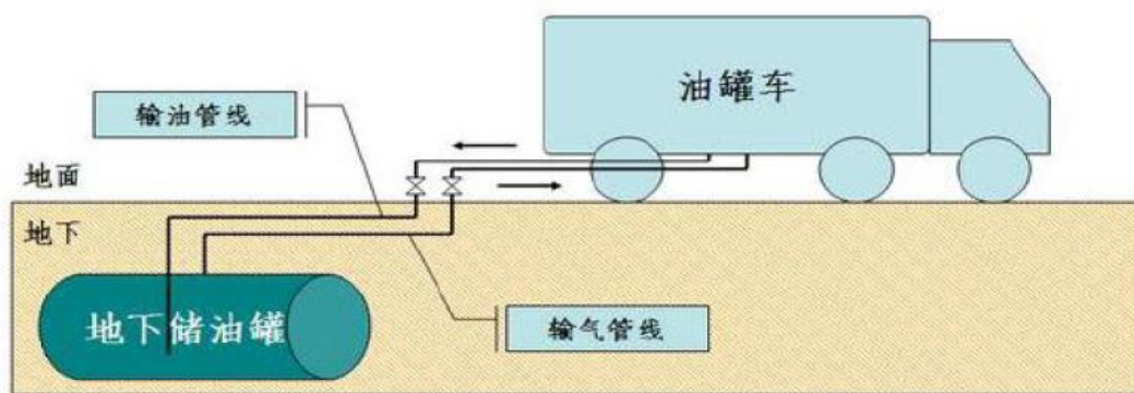
图 5-4 卸油油气回收工艺流程图
